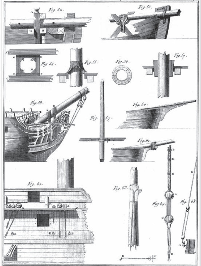
Traité de la Mâture pour les Elèves de la Marine. Pl. 7.
