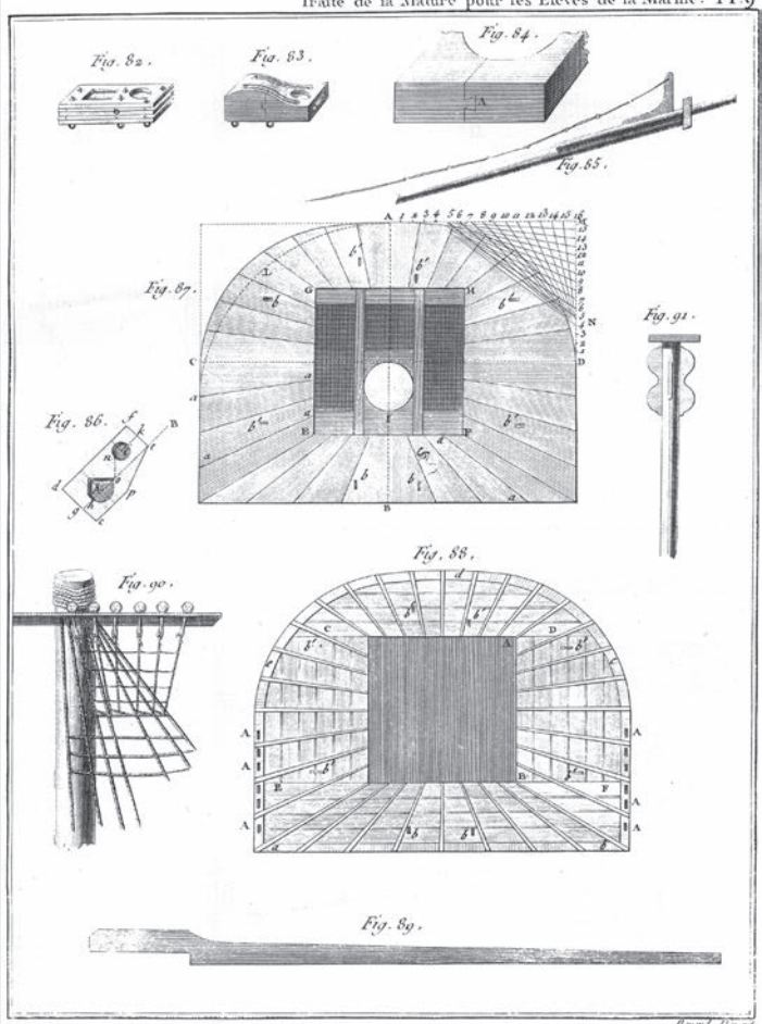
Traité de la Mâture pour les Elèves de la Marine. Pl. 9.
