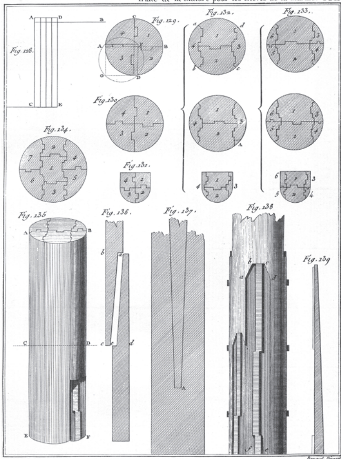
Traité de la Mâture pour les Elèves de la Marine. Pl. 5.
